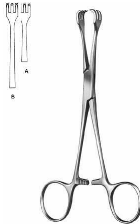
Lahey II-16-111-15 Goitre Grasping Forceps 15.5 cm
